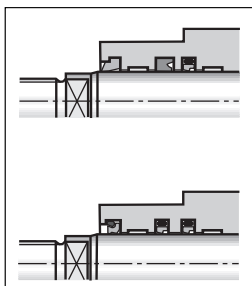
Piston rod
