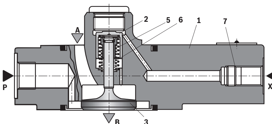
Type ZSF ... (NG32 ... 160)
