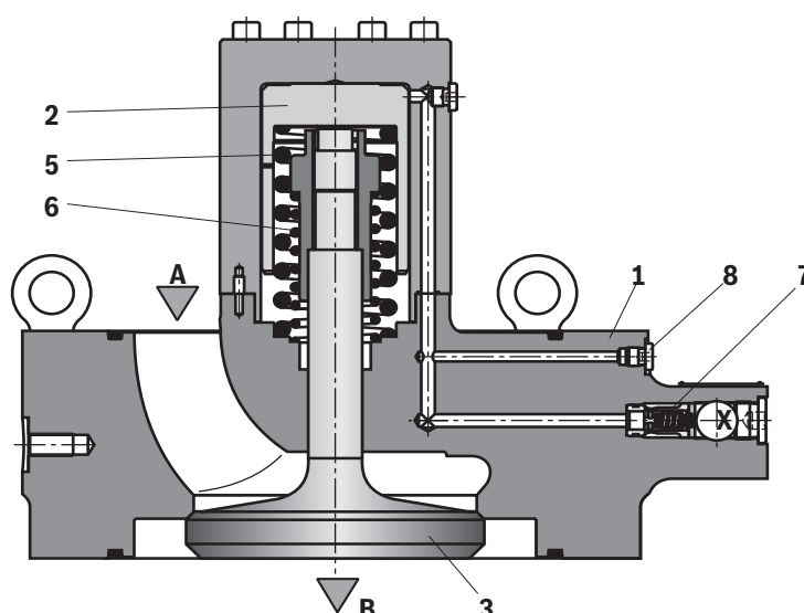
Type ZSF ... (NG200)
