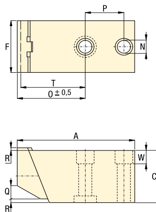
ECM-5, -20
