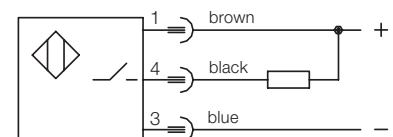
npn (-) switching
