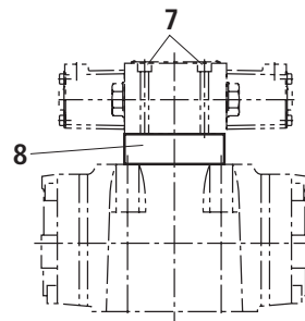
Type 4W.H 10 ..4X/.../...D3
