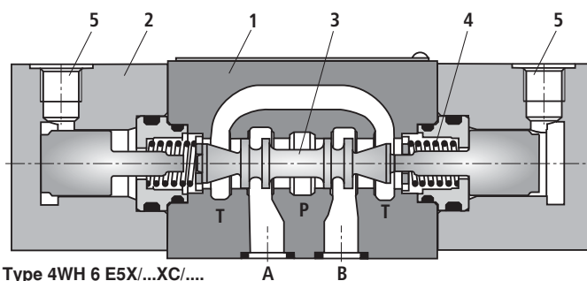
Type 4WH 6 E5X/...XC/...
