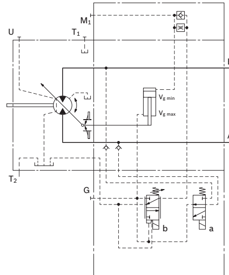
Schematic HA1R1, HA1R2
