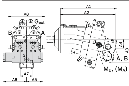
A6VM...HA
