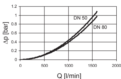
DF 2000, 3000, 4000
