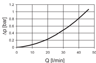
DF 60, 110, 140
