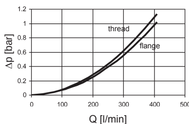
DF 160, 240, 280
