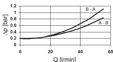
DFF 160, 240, 280
