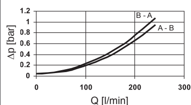
DFF 1500
