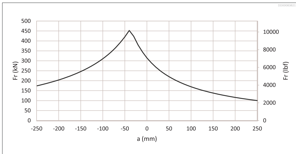
Fig. 38: Permissible external static load Häggglunds CAB 30 C (center flange)
