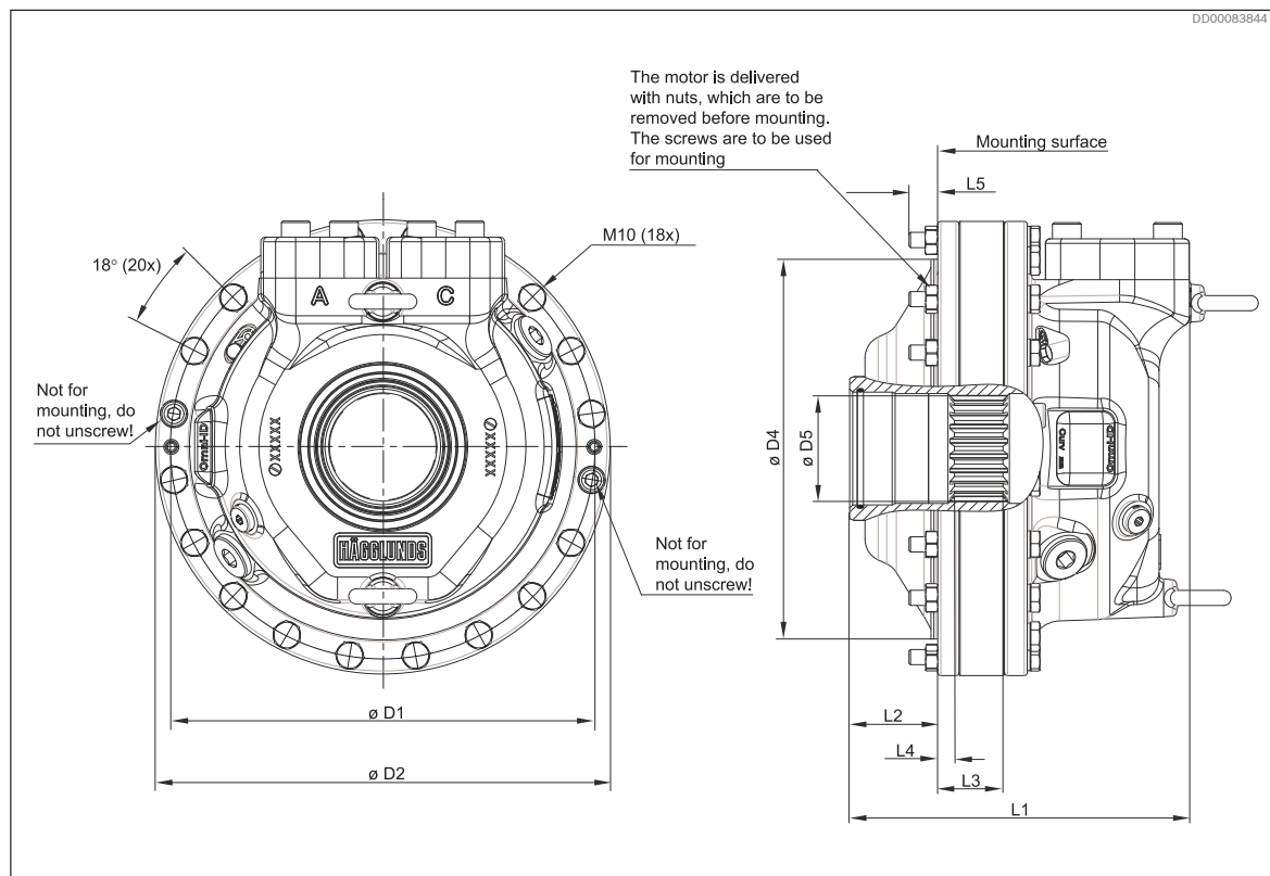
Fig. 42: CAb 10
