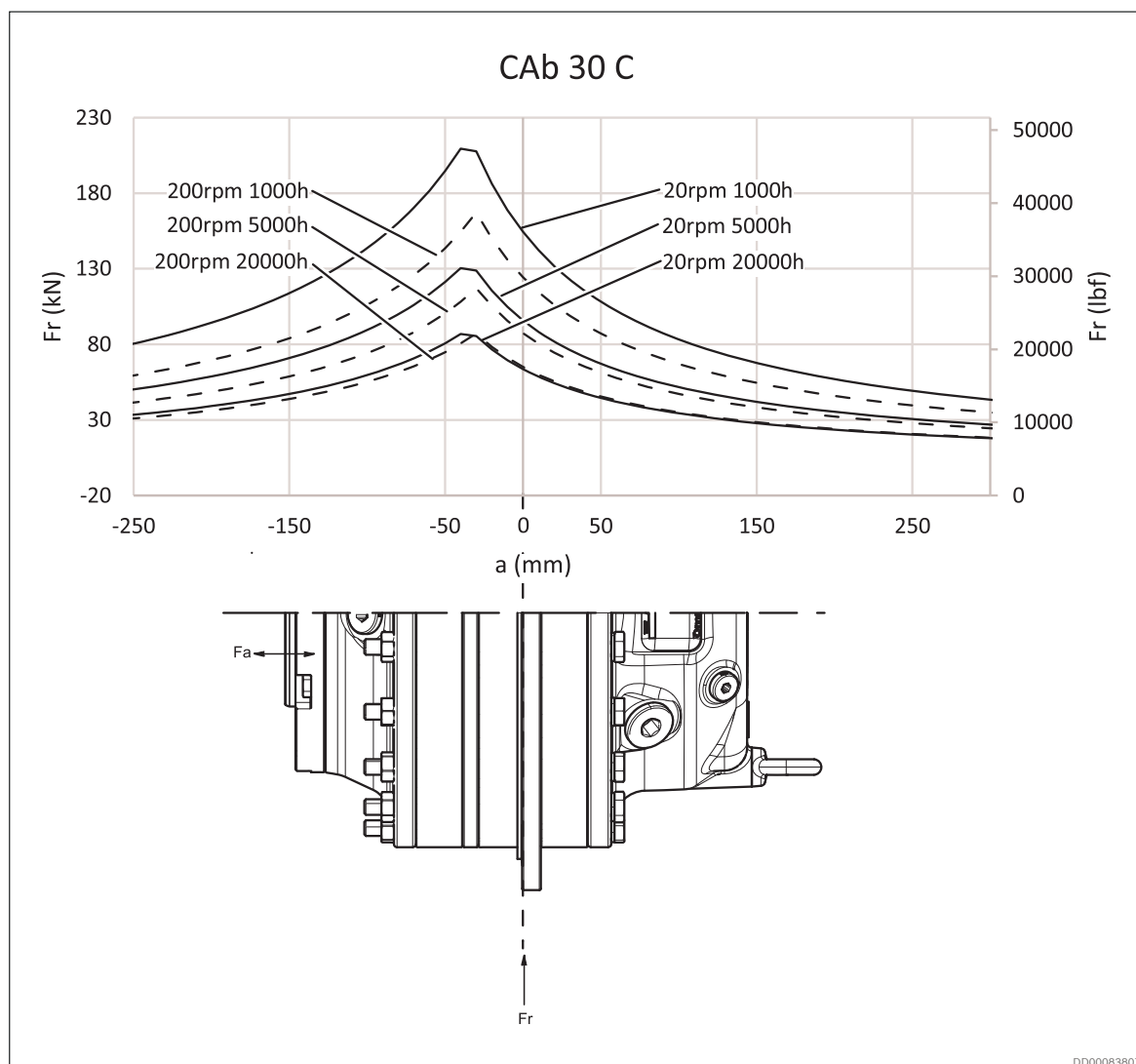
Fig. 33: Permissible external dynamic load Häggblunds CAB 30 C (center flange)
