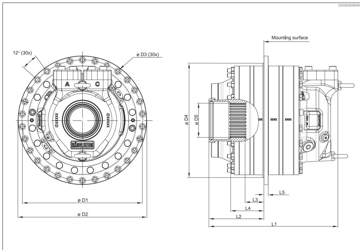
Fig. 46: CAB 40
