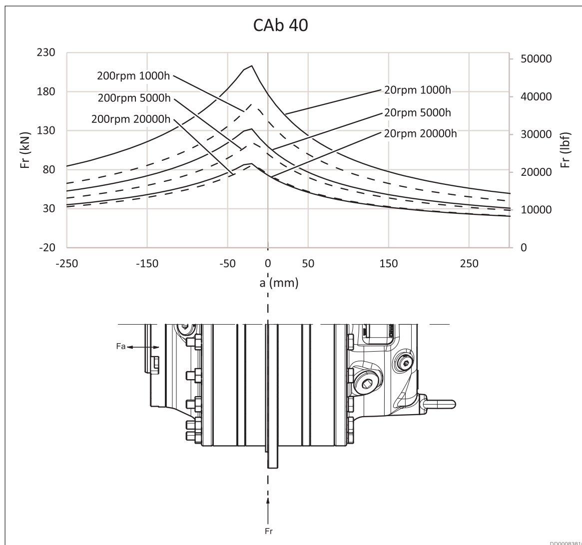
Fig. 35: Permissible external dynamic load Häggblunds CAb 40
