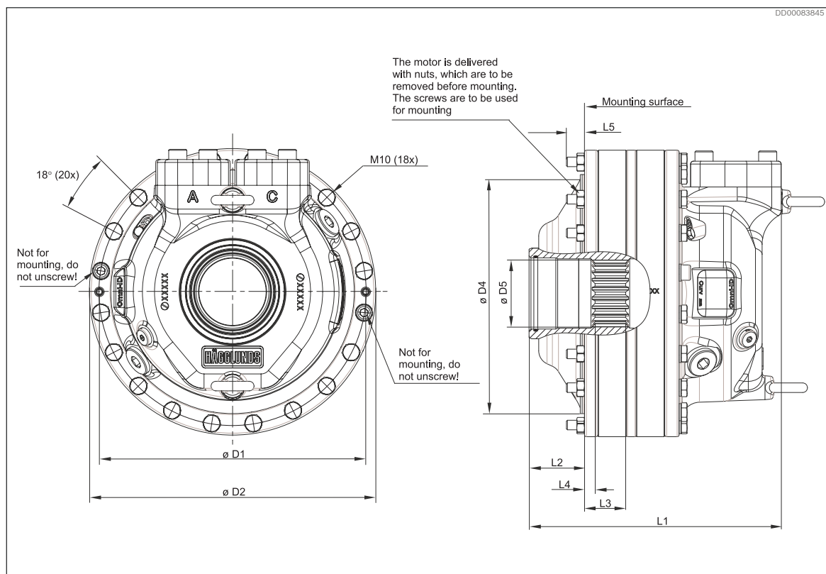
Fig. 43: CAb 20
