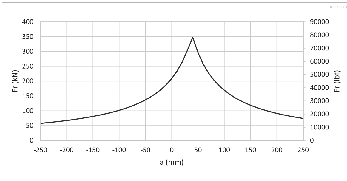
Fig. 36: Permissible external static load Häggblunds CAb 10
