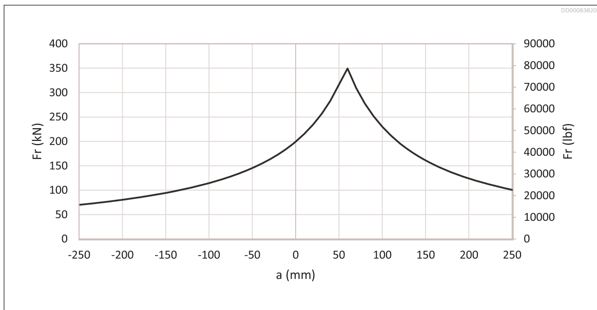
Fig. 37: Permissible external static load Häggblunds CAb 20
