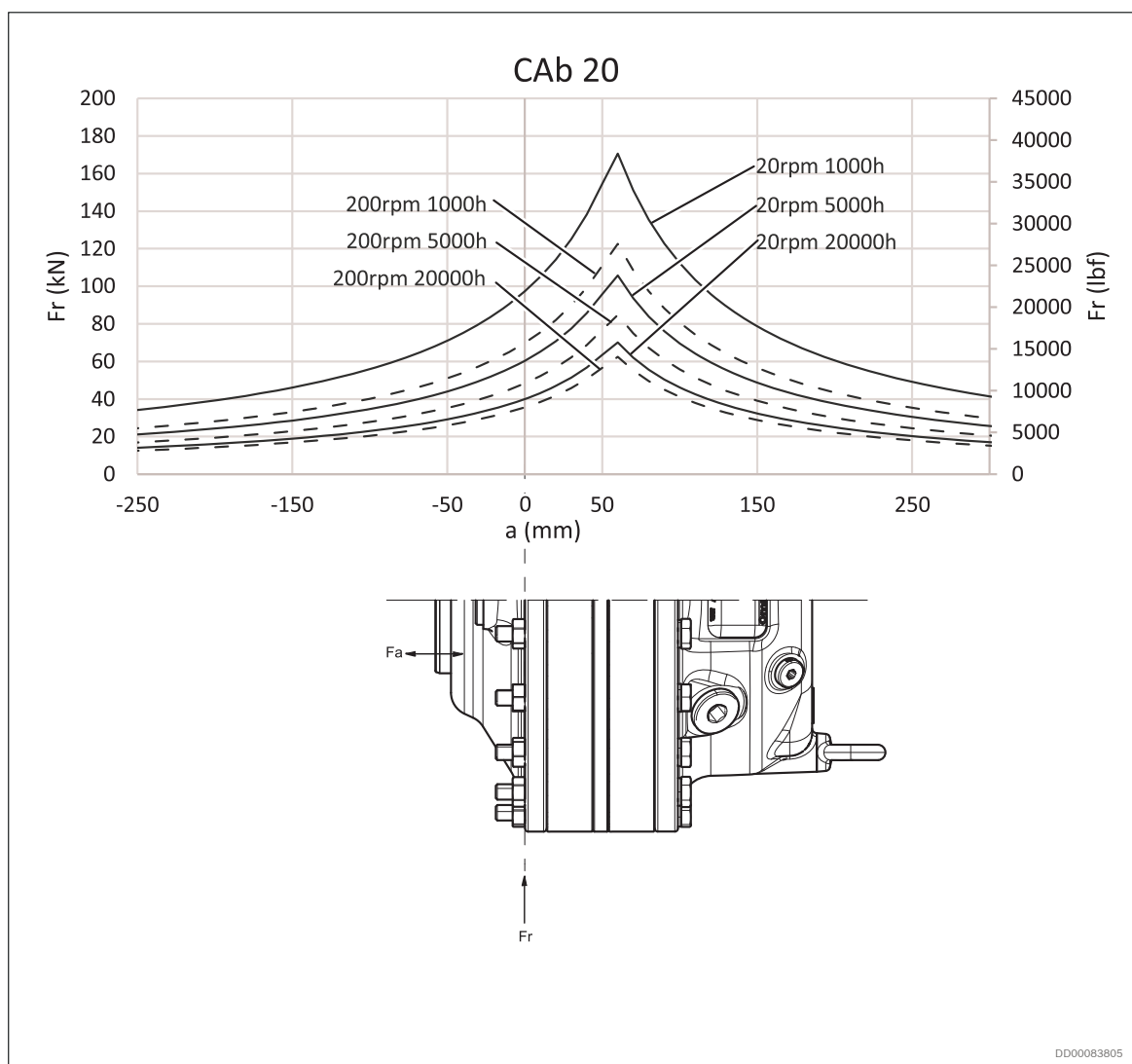
Fig. 32: Permissible external dynamic load Häggglunds CAb 20
