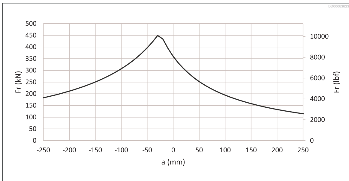
Fig. 40: Permissible external static load Häggglunds CAb 40
