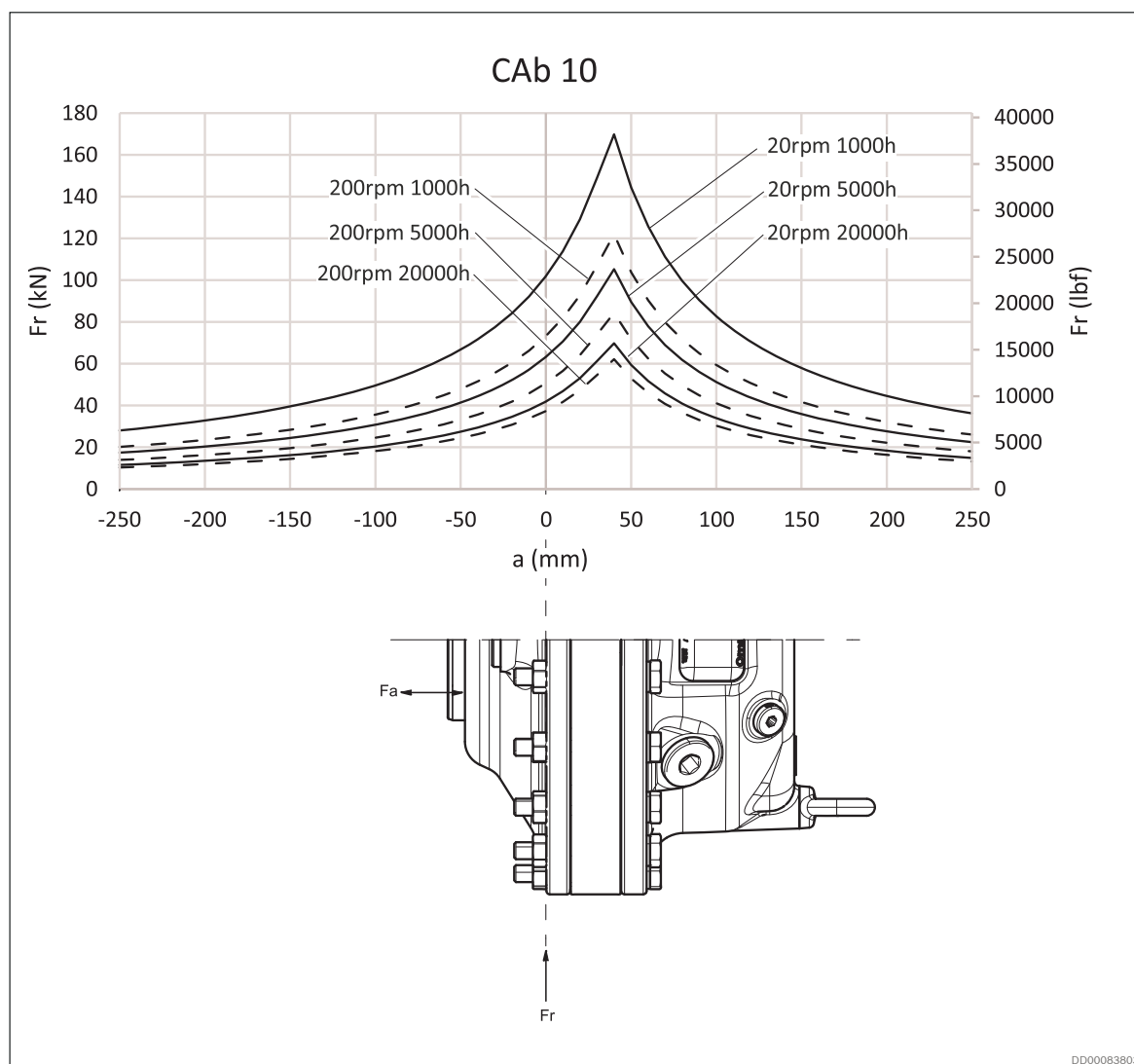
Fig. 31: Permissible external dynamic load Hägglunds CAB 10
