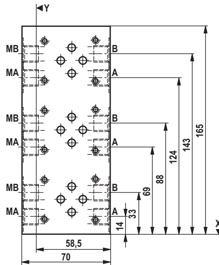
Dimensions
