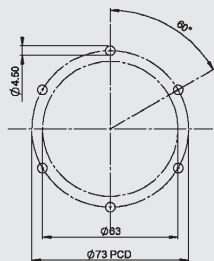
Interface to DIN 24557/Part 2
