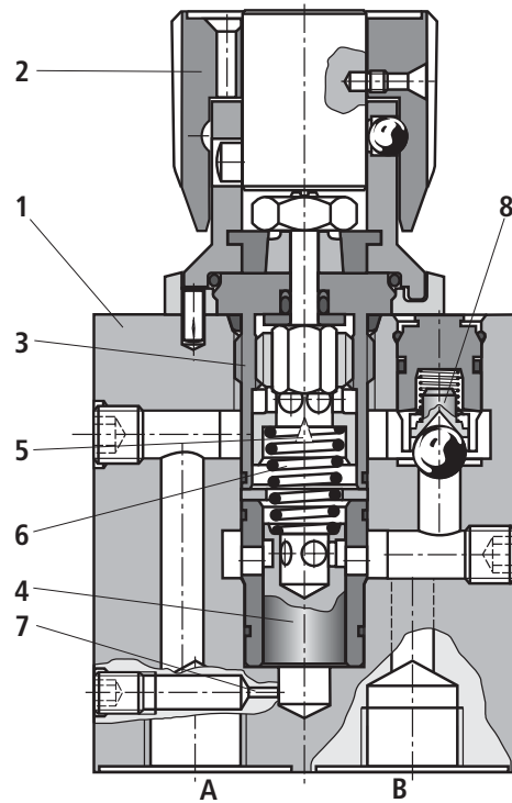
Type 2FRM 6 SB76-3X/..R...
