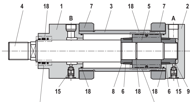
Piston rod
