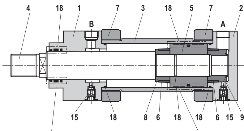
Piston rod
