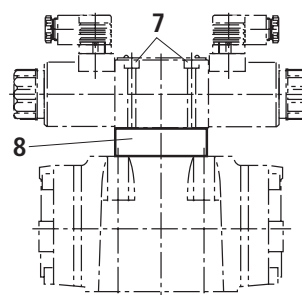
Type .WEH 10 ..4X/.../..D3
