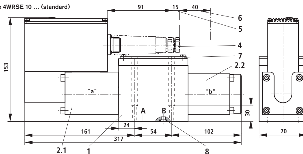
Type 4WRSE 10 C...
