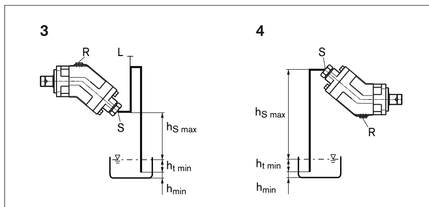
Abb. 9: Übertankeinbau mit Einbaulage 3–4
