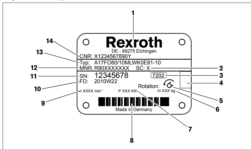
Abb. 4: Typschild A17FO
