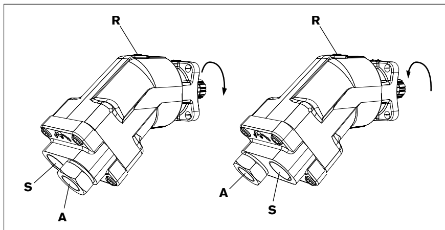
Abb. 13: Anschlussübersicht A17FO/A17FNO Baureihe 10
