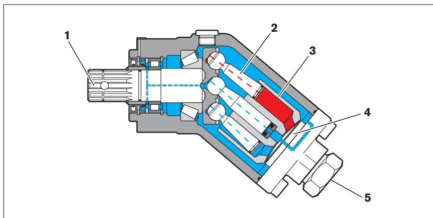
Abb. 2: Aufbau der A17FO/A17FNO Baureihe 10
