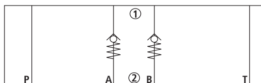
Type Z1S 6 C ...
