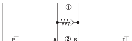
Type Z1S 6 B-A ...
