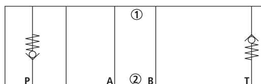
Type Z1S 6 F ...
