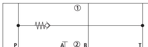
Type Z1S 6 T-P ...
