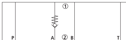
Type Z1S 6 P ...
