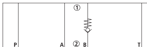
Type Z1S 6 T ...
