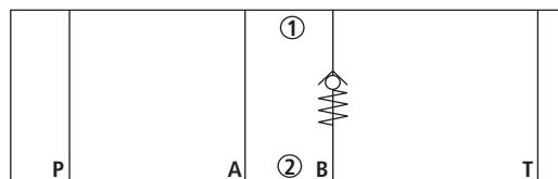
Type Z1S 6 B ...
