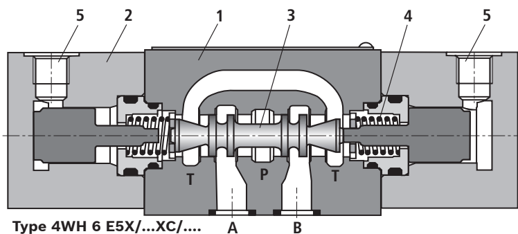
Type 4WH 6 E5X/...XC/...
