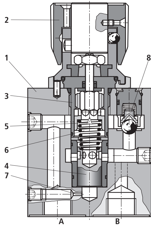
Type 2FRM 6 SB76-3X/..R...
