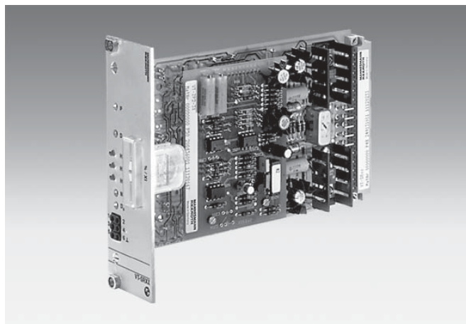
Type VT-SR7-1X/...
