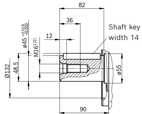
B1 – Ø45 A 14x9x80
