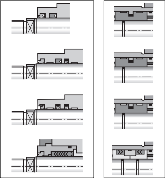
Piston rod
